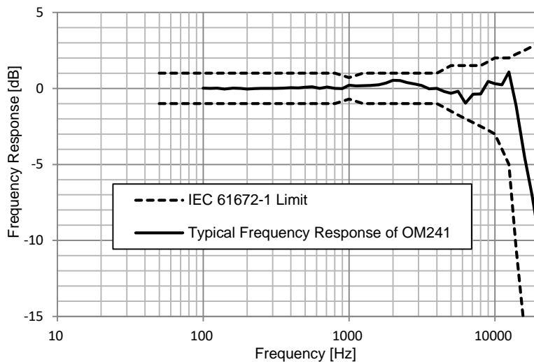
OM241 典型 0 度入射自由场频率响应
