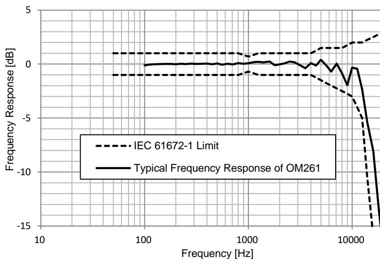
OM261 典型 90 度入射自由场频率响应
